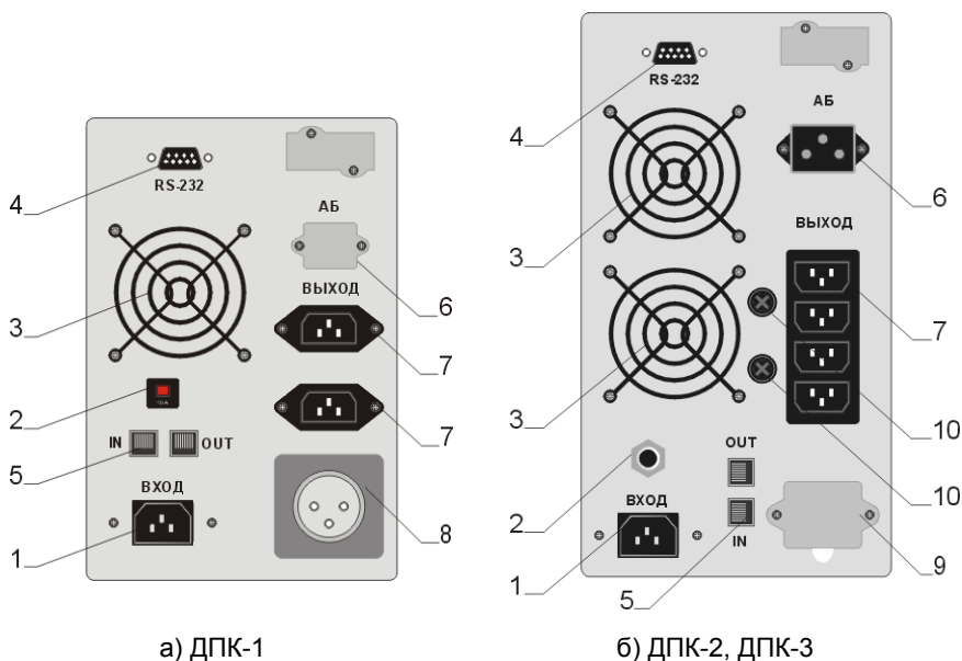
Рис. 2 Задняя панель блока ИБП:
