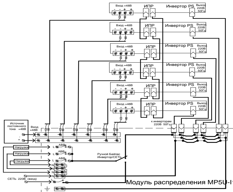
Типовая схема соединений с использованием 5U модуля распределения МР5U-11 с применением БАЙПАСА мощностью до 9 кВт.
